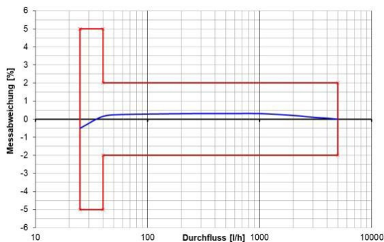
Typische Fehlerkurve für Q 3 4 R160H
